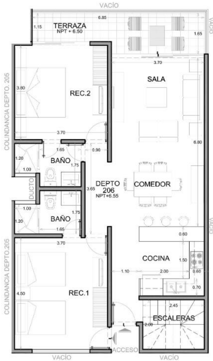
PLANTA ARQUITECTÓNICA ESC. 1:100
